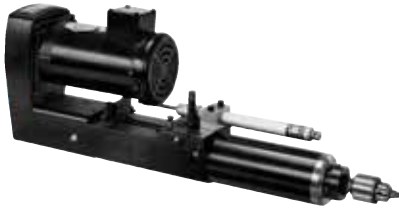
Elektro-Pnömatik İlerlemeli Otomatik Delik Delme Ünitesi
