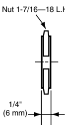
39476 Nut 1-7/16—18 L.H. Thread
